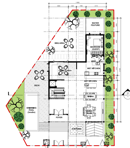
TẦNG TRỆT Level 1 156 SQM
