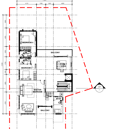
TẦNG 2 Level 2 156 SQM
