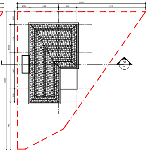
TẦNG MÁI Proof plan
