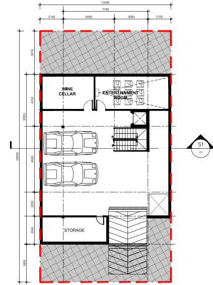
TẦNG HẦM sub-basement 173 SQM
