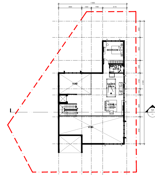
TẦNG LỬNG Mezzanine 93 SQM
