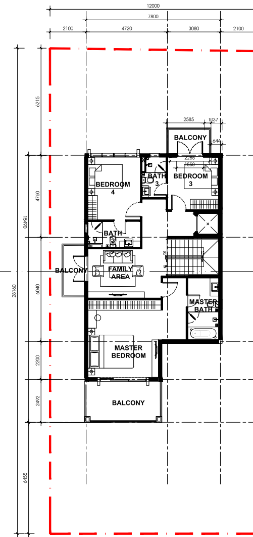
TẦNG 2 Level 2 98 SQM
