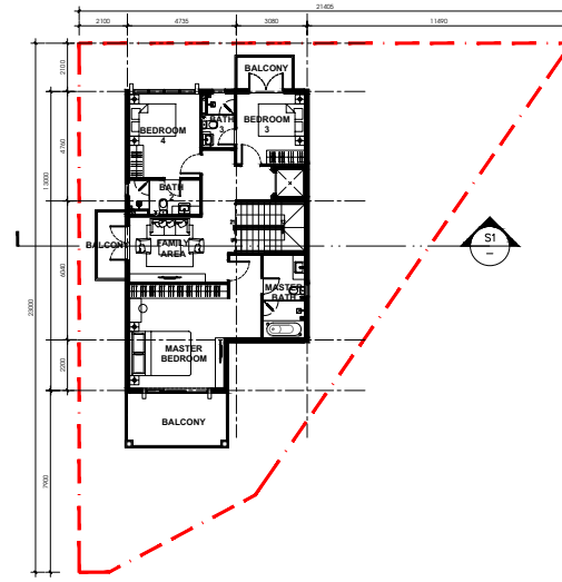
TẦNG 2 Level 2 98 SQM
