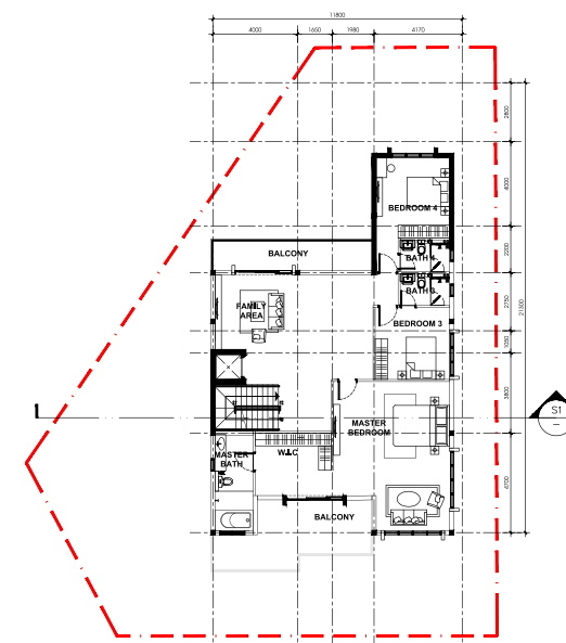
TẦNG 2 Level 2 156 SQM
