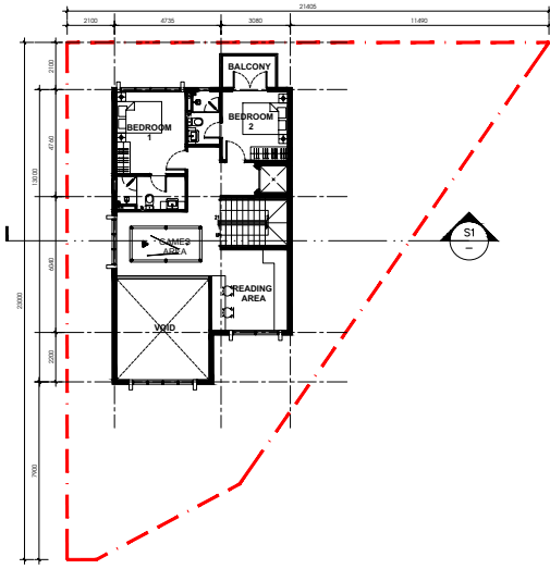
TẦNG LỬNG Mezzanine 79 SQM
