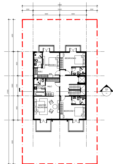
TẦNG 2 Level 2 128 SQM
