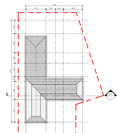
TẦNG MÁI Proof plan
