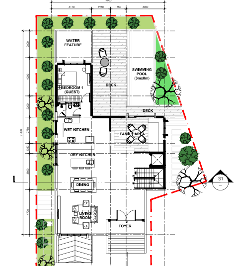
TẦNG TRỆT Level 1 156 SQM
