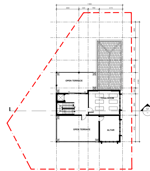
TẦNG 3 Level 3 68 SQM
