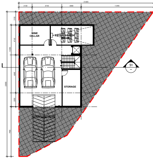
TẦNG HẦM sub-basement 130 SQM
