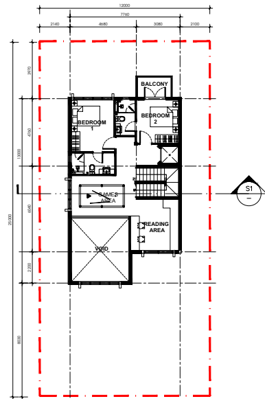
TẦNG LŨNG Mezzanine 79 SQM
