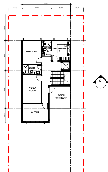
TẦNG 3 Level 3 85 SQM
