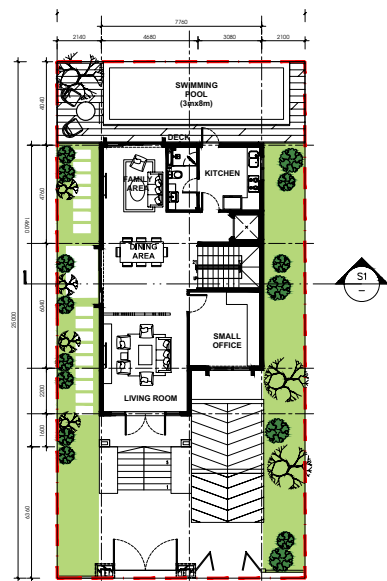
TẦNG TRỆT Level 1 98 SQM
