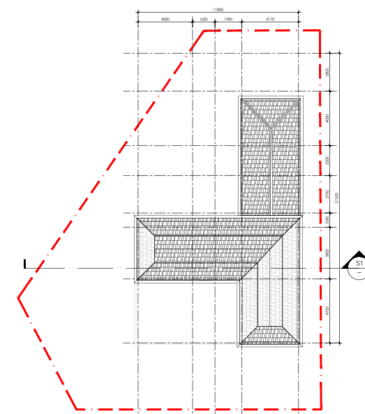
TẦNG MÁI Proof plan
