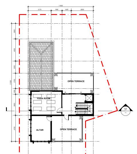
TẦNG 3 Level 3 68 SQM
