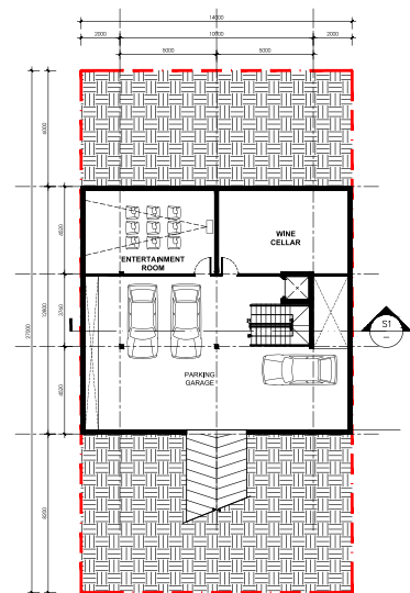
TẦNG HẦM sub-basement 179 SQM
