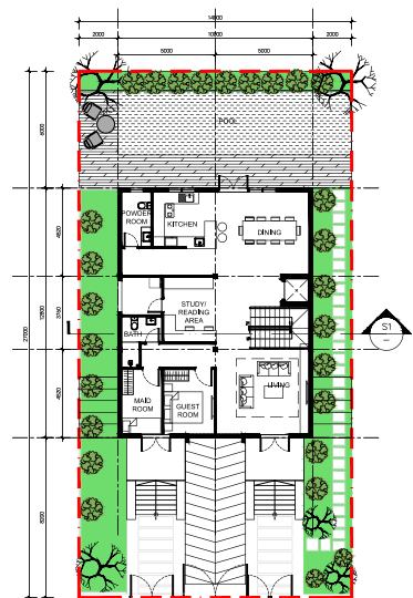
TẦNG TRỆT Level 1 128 SQM
