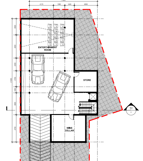
TẦNG HẦM sub-basement 237 SQM
