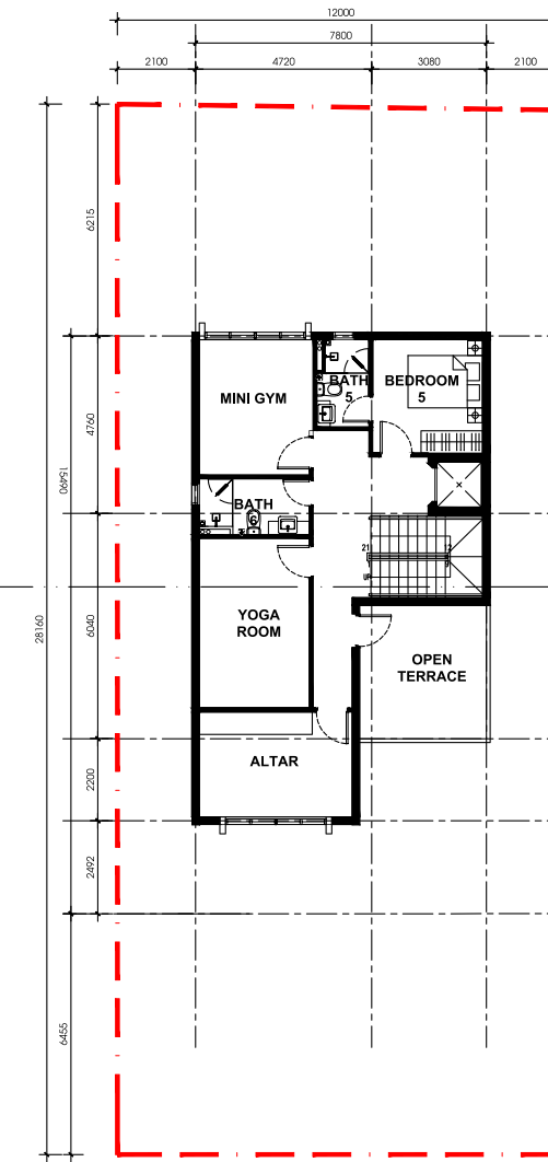
TẦNG 3 Level 3 85 SQM
