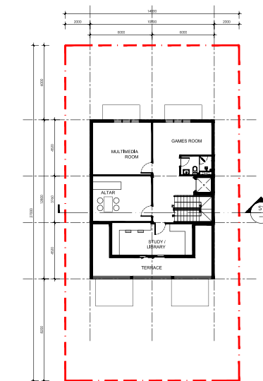
TẦNG 3 Level 3 102 SQM
