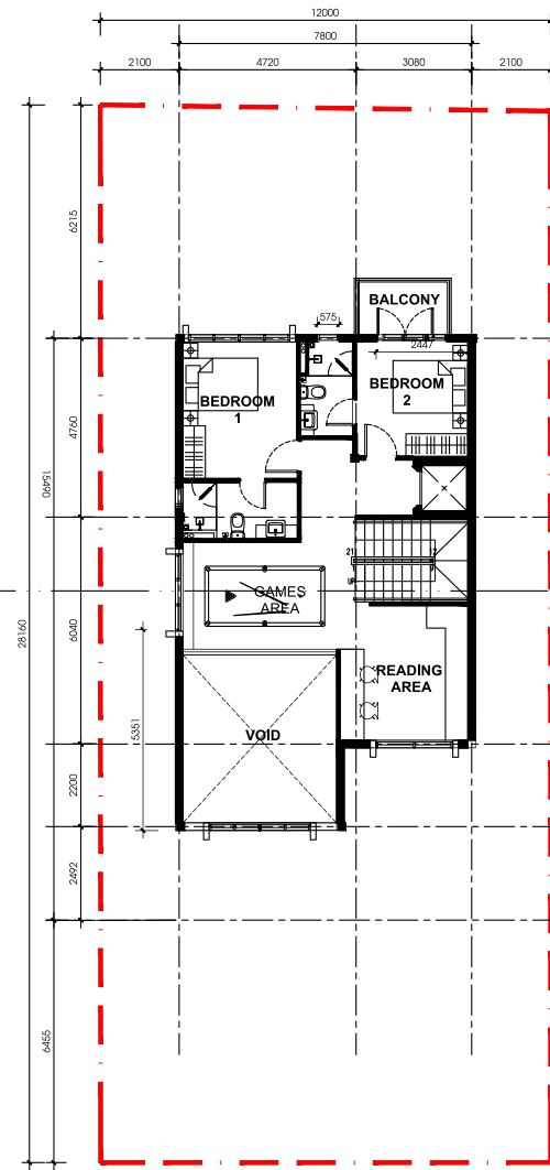
TẦNG LỬNG Mezzanine 79 SQM
