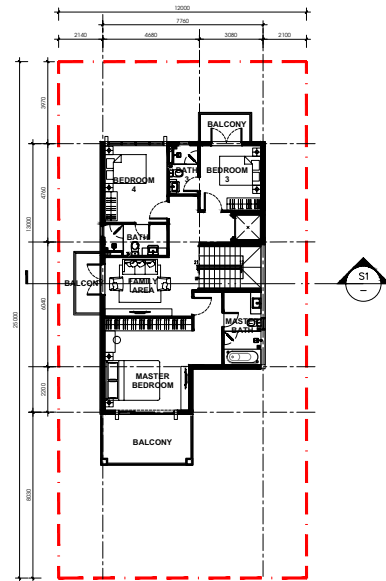
TẦNG 2 Level 2 98 SQM
