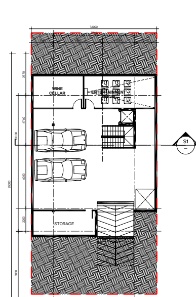
TẦNG HẦM sub-basement 173 SQM
