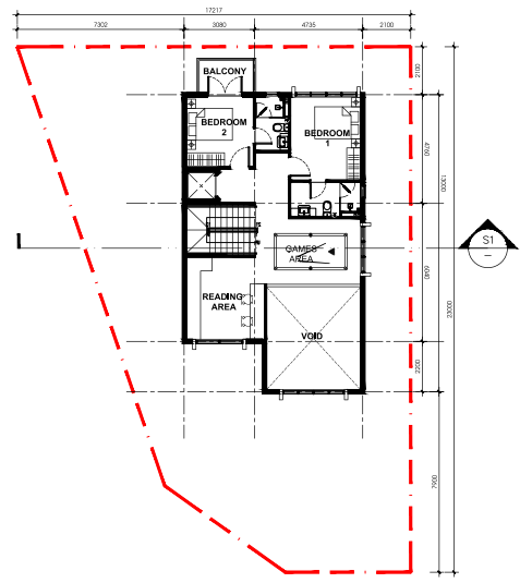
TẦNG LỬNG Mezzanine 79 SQM
