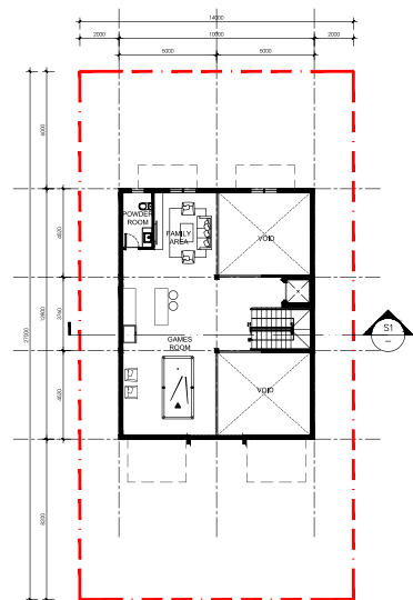
TẦNG LỬNG Mezzanine 88 SQM
