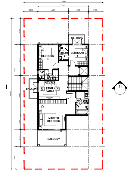
TẦNG 2 Level 2 98 SQM
