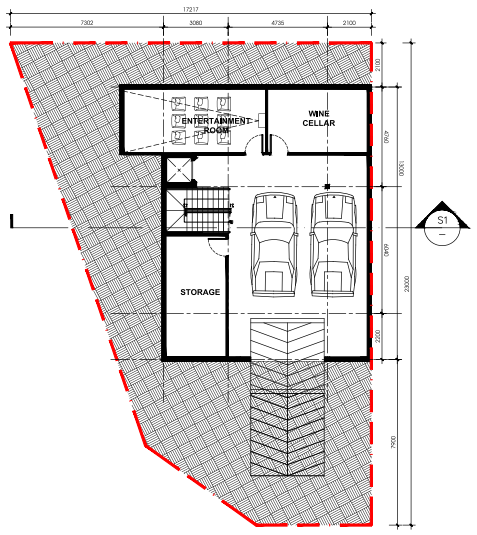
TẦNG HẦM sub-basement 138 SQM
