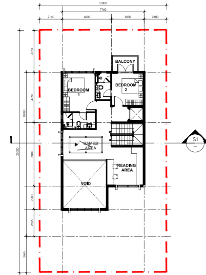
TẦNG LỬNG Mezzanine 79 SQM
